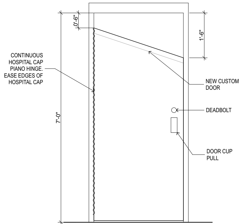
TYP. DOOR MODIFICATION
